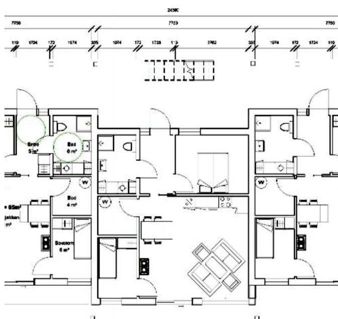
Plantegning Stuslåtta 3 nede, 3b er i midten.
